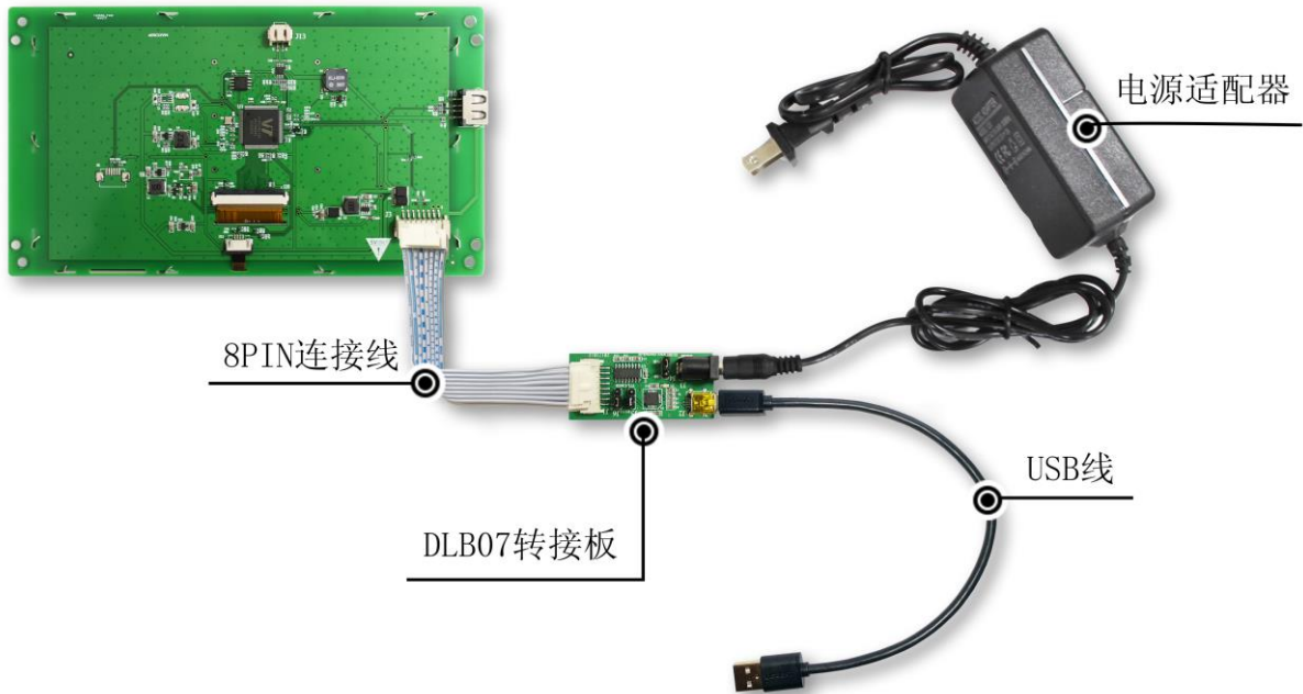
图 3 转接板 DLB07 与串口屏的连接
