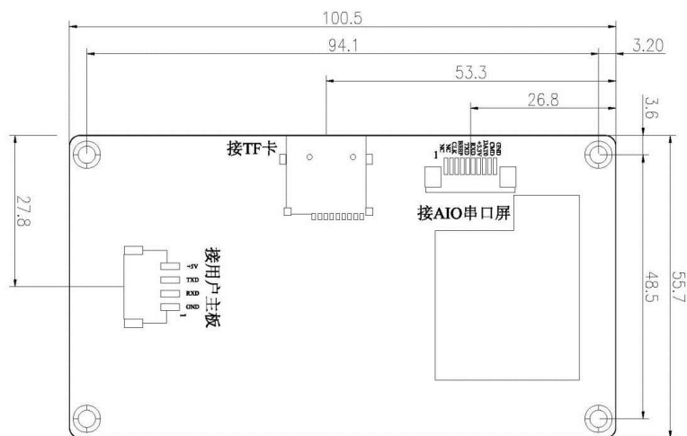
图 8 转接板 AIO035-A 尺寸图
