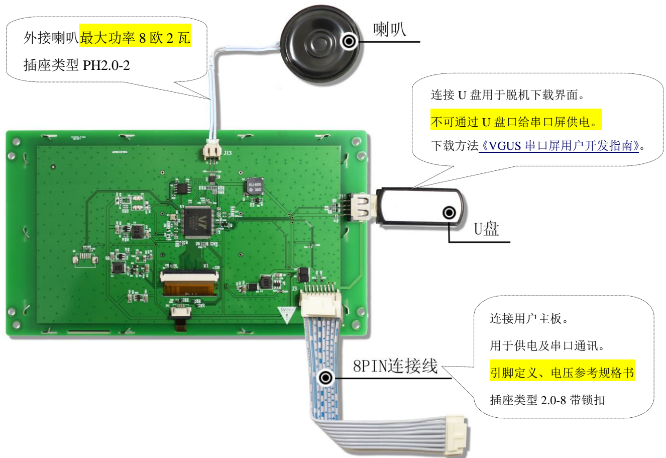
图 1 SDWa070C03T 外部接口连接示意图
