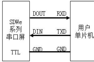
图 2A TTL 接口
