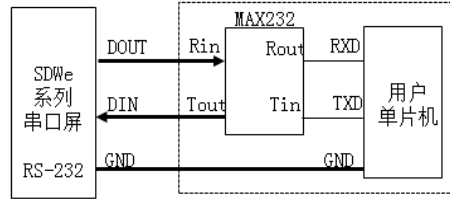
图 2B RS-232 接口
