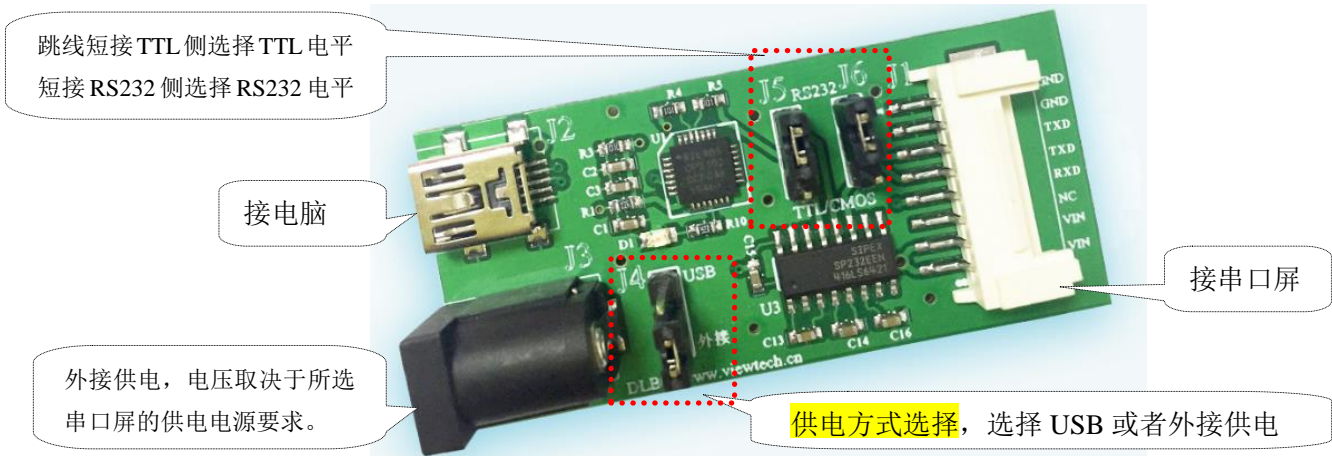
图 12 转接板 DLB07 实物图
