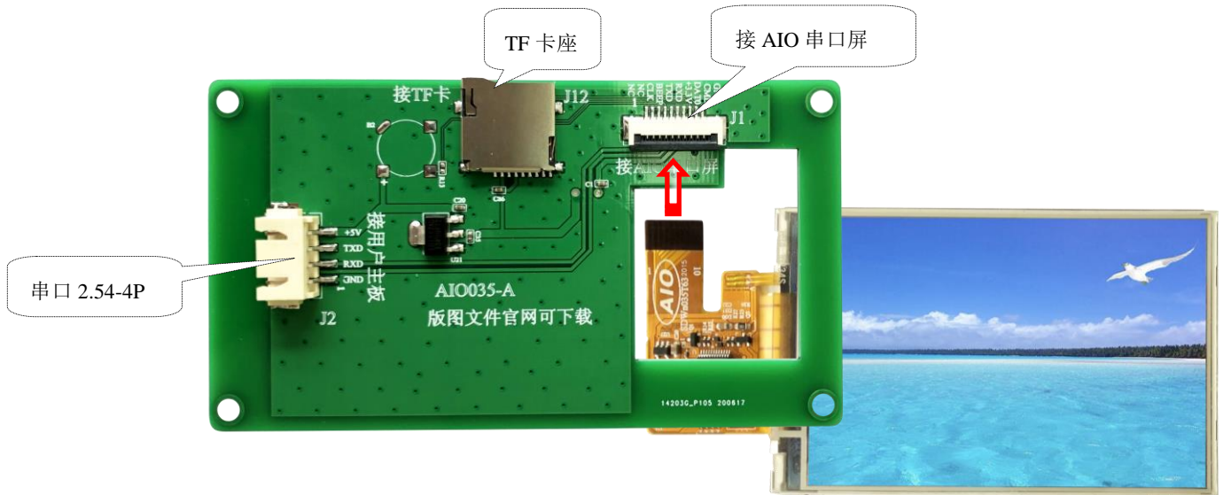
图 9 转接板 AIO035-A
