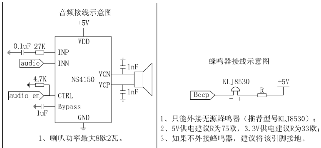
图 4 喇叭与蜂鸣器应用电路
