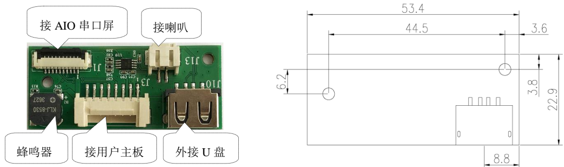
图 6 转接板 AIO03
