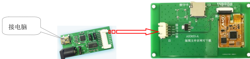
图 11 DLB07 与转接板 AIO035 连接示意图
