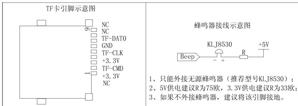
图 7 TF 卡与蜂鸣器应用电路
