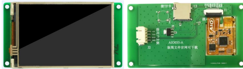
图 10 转接板 AIO035-A 与串口屏粘贴后示意图
